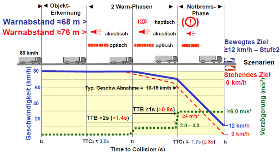
Bild 2: Kollisionswarn- und Bremsphasen aktuell-optimaler Notbrens-Assistenzsysteme für Güter-Kfz >8 t zGG mit Kollisionsvermeidbarkeit auch bei stehenden Objekten
