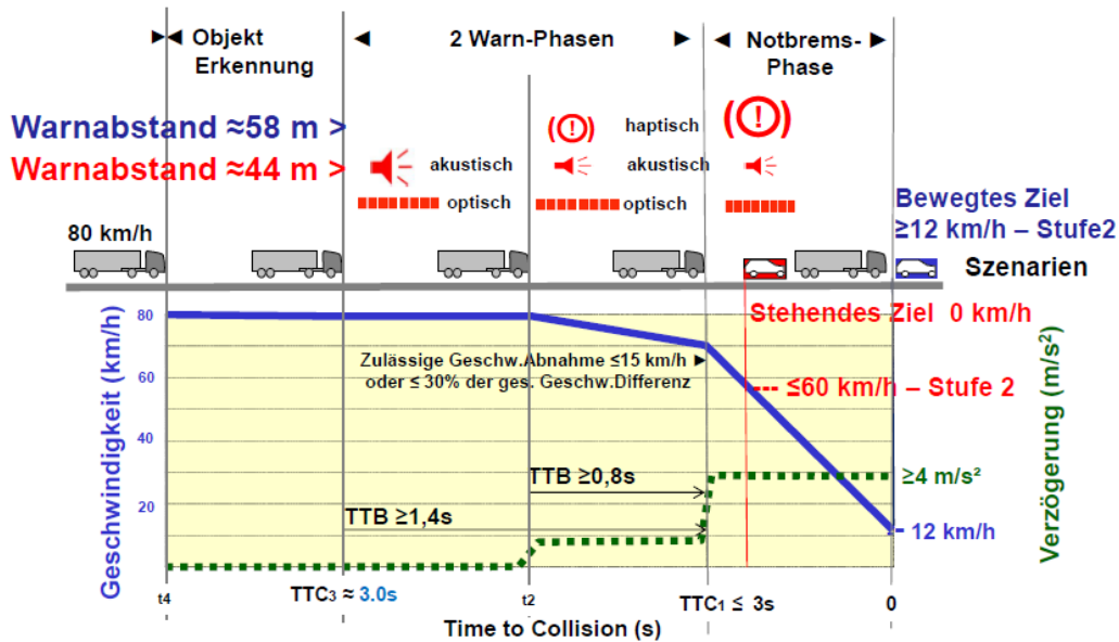
Bild 1: Kollisionswarn- und Bremsphasen aktueller Notbrens-Assistenzsysteme für Güter-Kfz >8 t zGG gemäß EU-Verordnung 347/2012/EC, Anforderungsstufe 2 – vor langsamem oder stehendem Objekt
